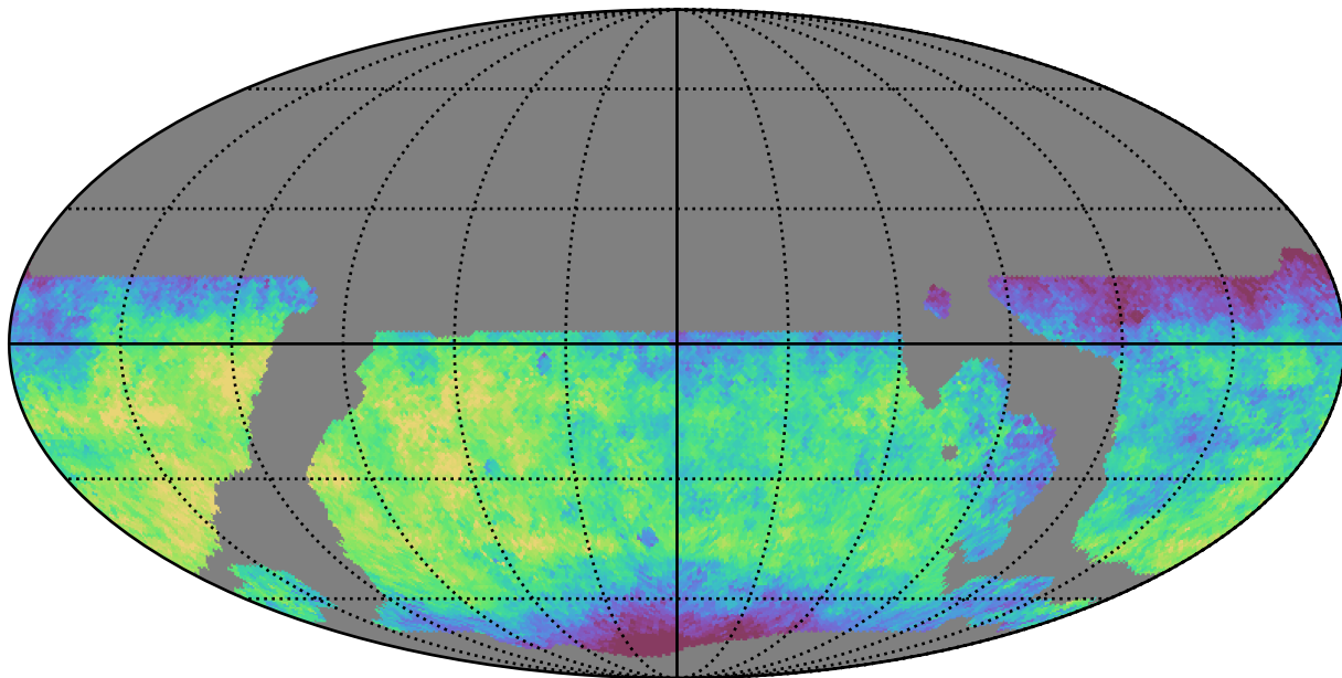
weather_cloudso14v3.4_10yrs WFD y band: Median saturation_mag
