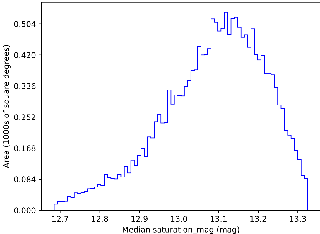
weather_cloudso14v3.4_10yrs WFD y band: Median saturation_mag
