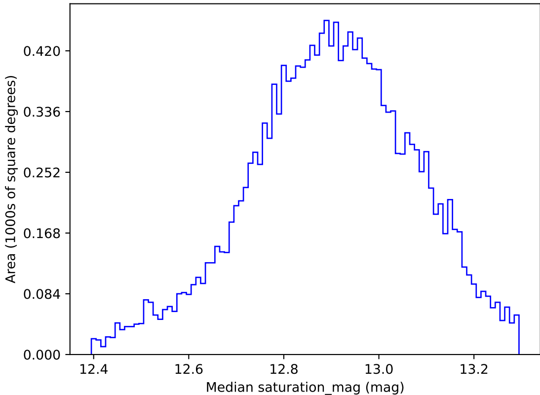
weather_cloudso14v3.4_10yrs WFD u band: Median saturation_mag
