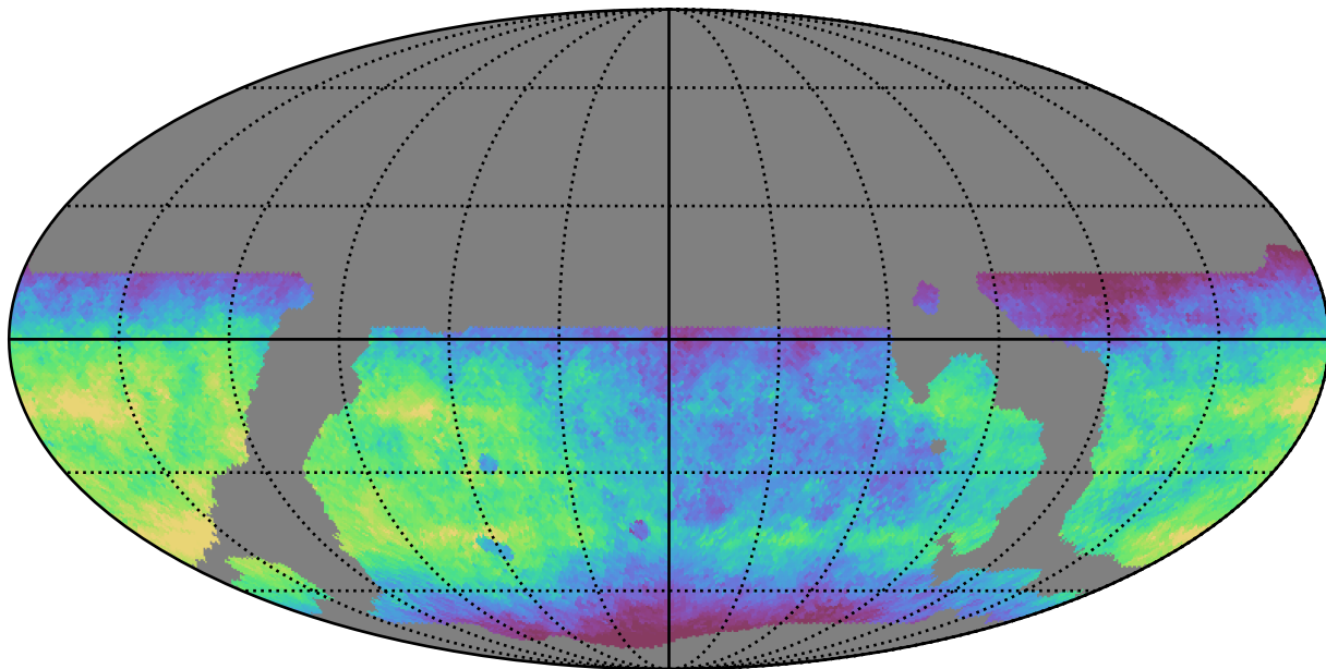
weather_cloudso14v3.4_10yrs WFD r band: Median saturation_mag
