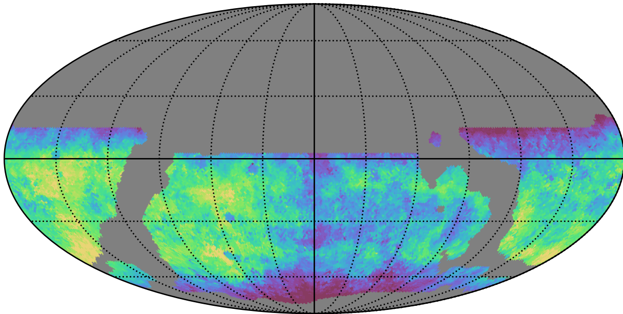
weather_cloudso14v3.4_10yrs WFD g band: Median saturation_mag
