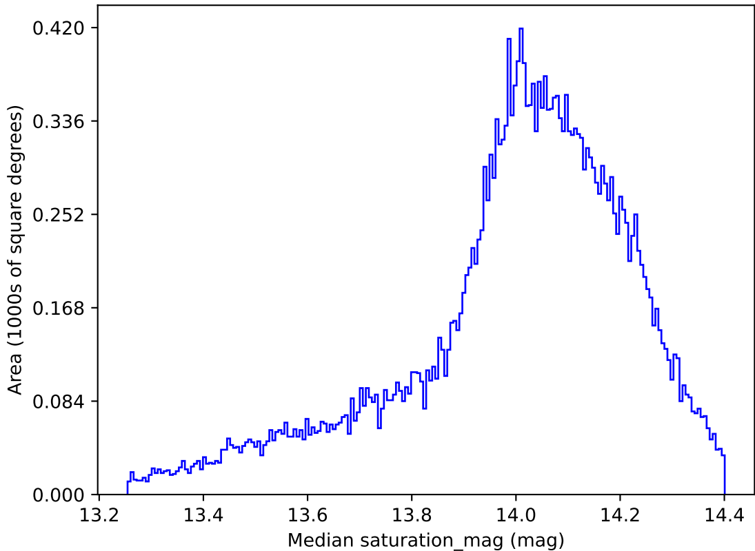
weather_cloudso14v3.4_10yrs All sky z band: Median saturation_mag
