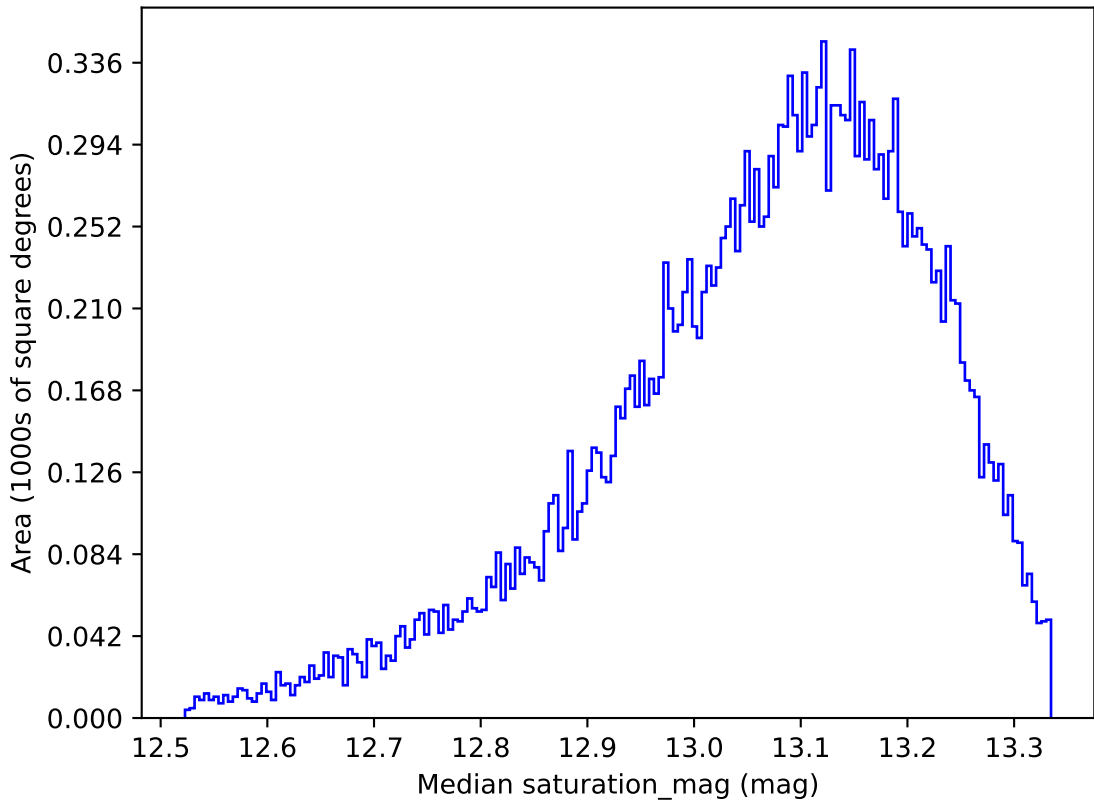
weather_cloudso14v3.4_10yrs All sky y band: Median saturation_mag
