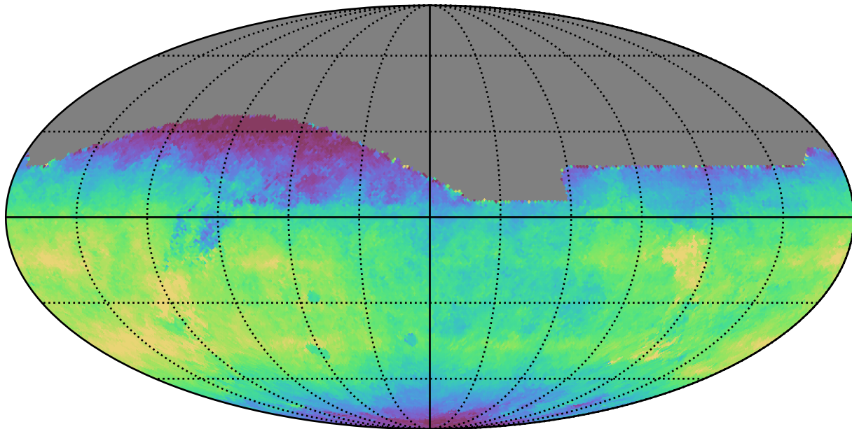
weather_cloudso14v3.4_10yrs All sky r band: Median saturation_mag
