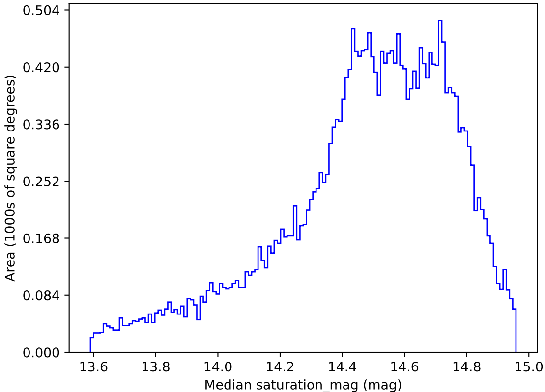
weather_cloudso14v3.4_10yrs All sky r band: Median saturation_mag
