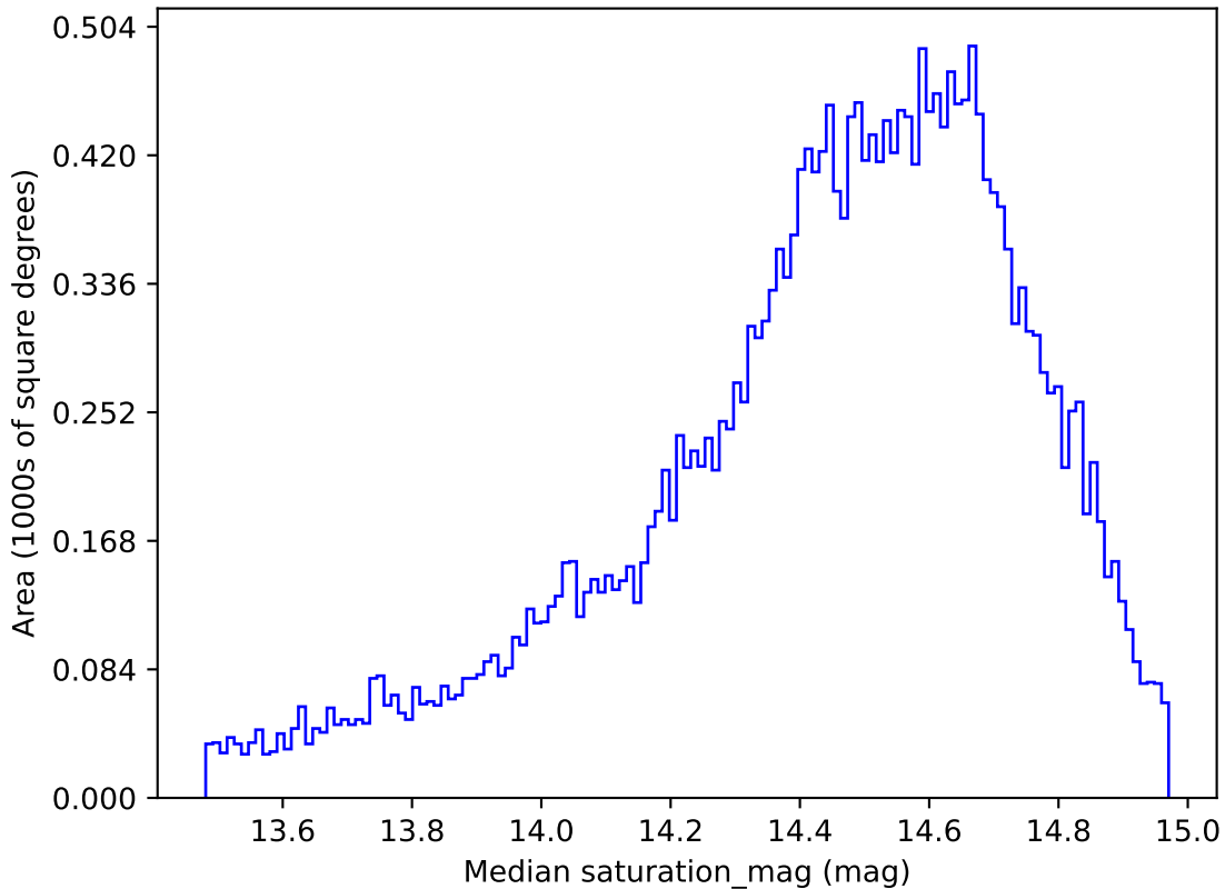
weather_cloudso14v3.4_10yrs All sky g band: Median saturation_mag
