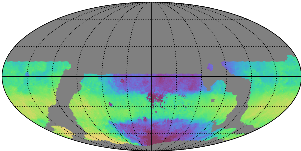
weather_cloudso14v3.4_10yrs WFD y band: Median HA
