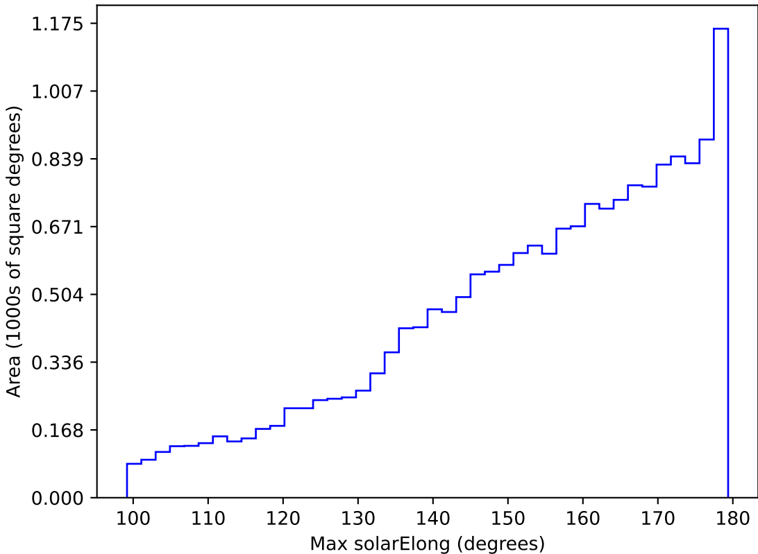
weather_cloudso14v3.4_10yrs WFD z band: Max solarElong
