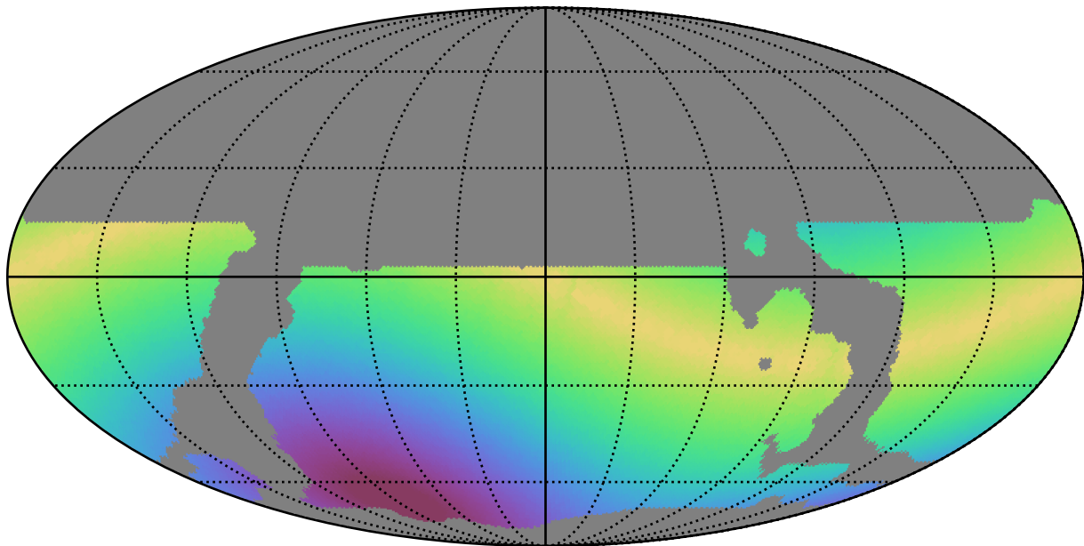
weather_cloudso14v3.4_10yrs WFD y band: Max solarElong
