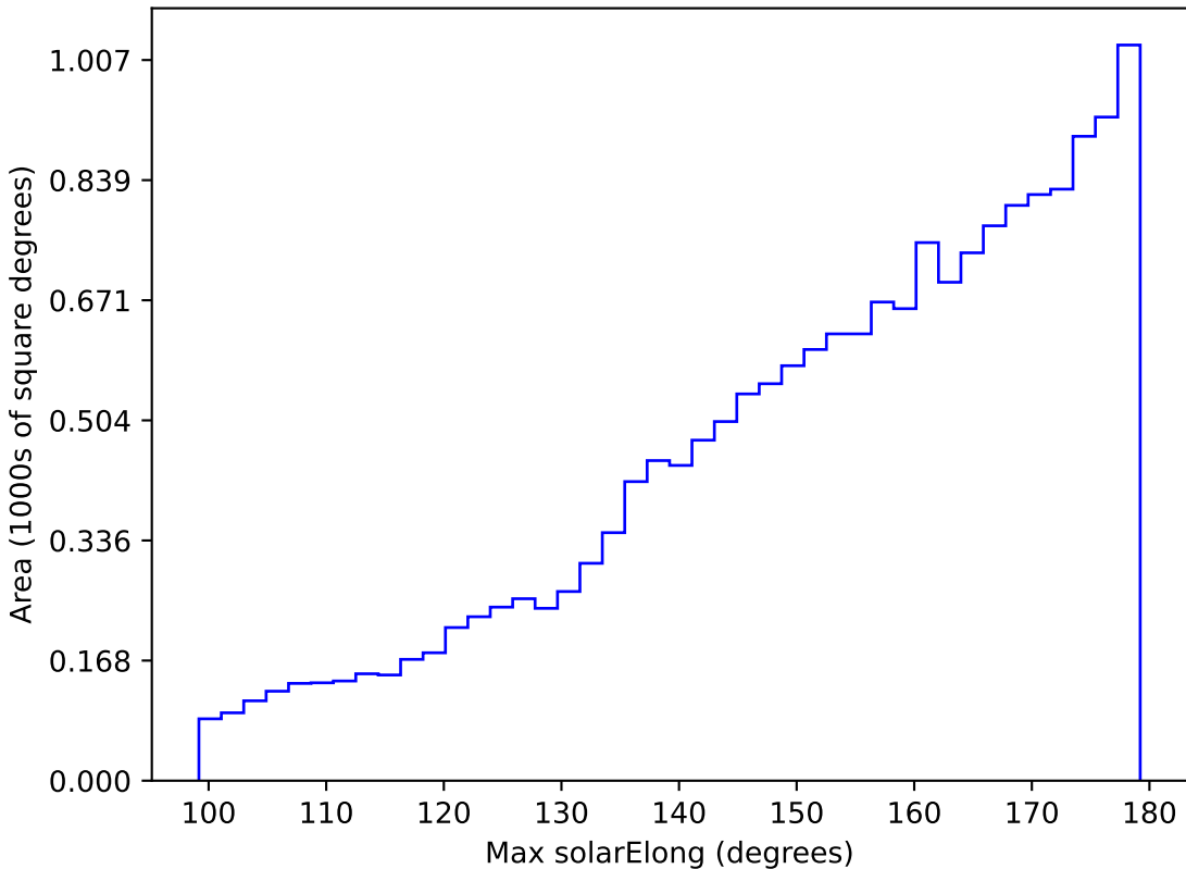
weather_cloudso14v3.4_10yrs WFD y band: Max solarElong
