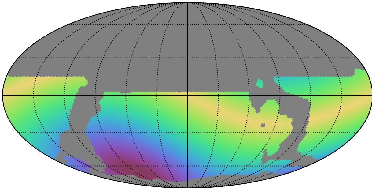
weather_cloudso14v3.4_10yrs WFD i band: Max solarElong
