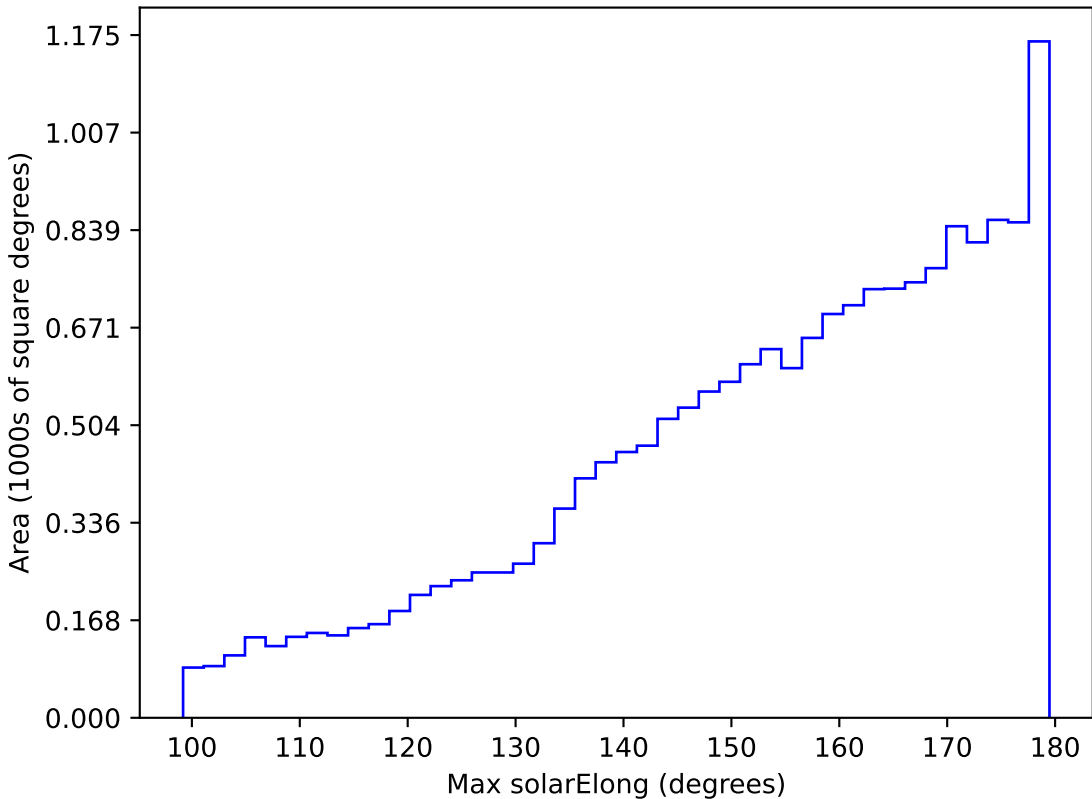
weather_cloudso14v3.4_10yrs WFD i band: Max solarElong
