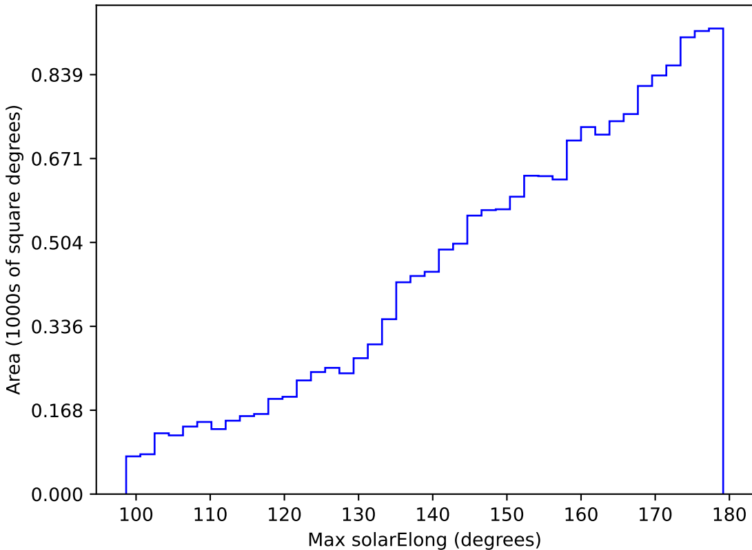
weather_cloudso14v3.4_10yrs WFD g band: Max solarElong
