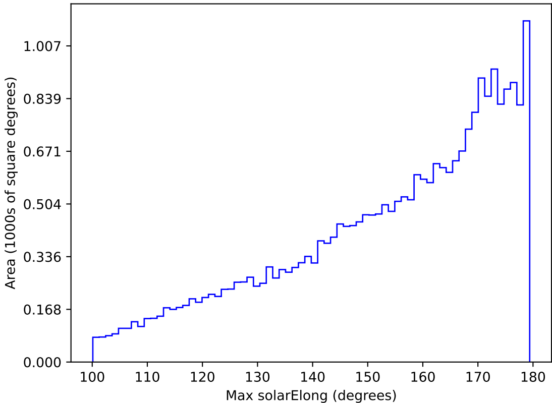
weather_cloudso14v3.4_10yrs All sky i band: Max solarElong
