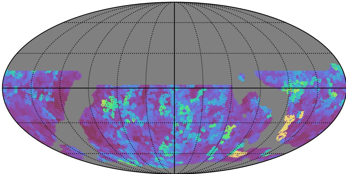
weather_cloudso14v3.4_10yrs WFD y band: Max seeingEff
