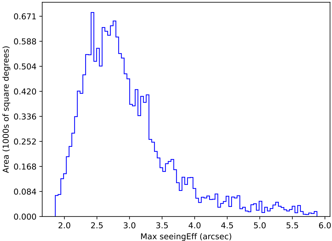
weather_cloudso14v3.4_10yrs WFD i band: Max seeingEff
