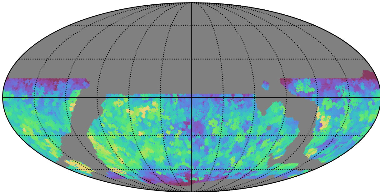
weather_cloudso14v3.4_10yrs WFD z band: Max saturation_mag
