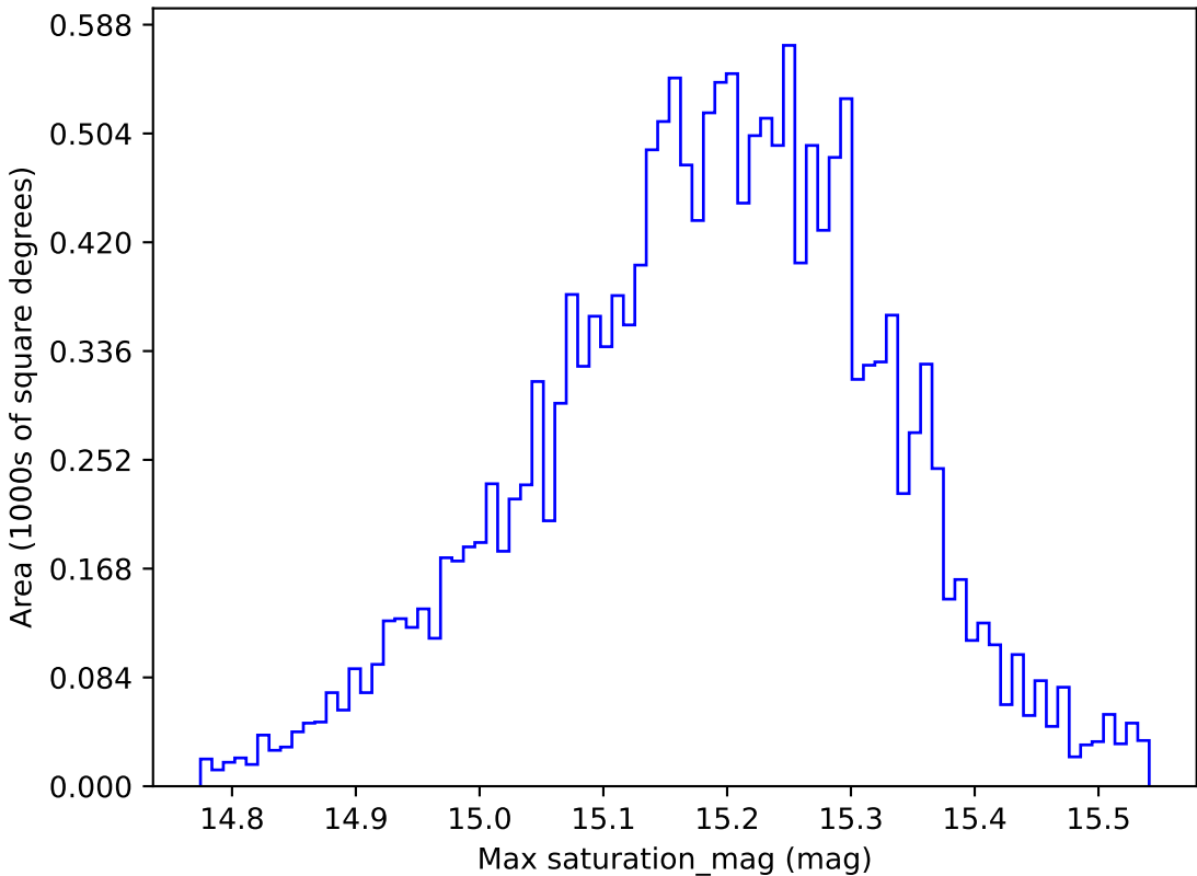
weather_cloudso14v3.4_10yrs WFD z band: Max saturation_mag
