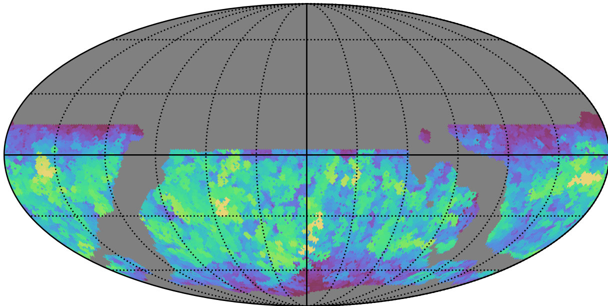
weather_cloudso14v3.4_10yrs WFD y band: Max saturation_mag
