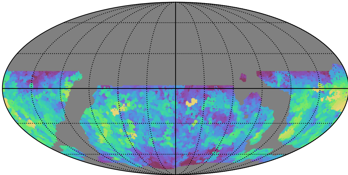
weather_cloudso14v3.4_10yrs WFD u band: Max saturation_mag
