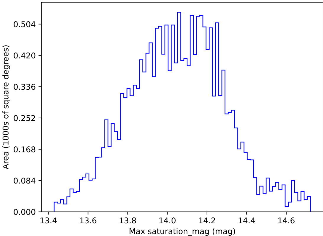
weather_cloudso14v3.4_10yrs WFD u band: Max saturation_mag
