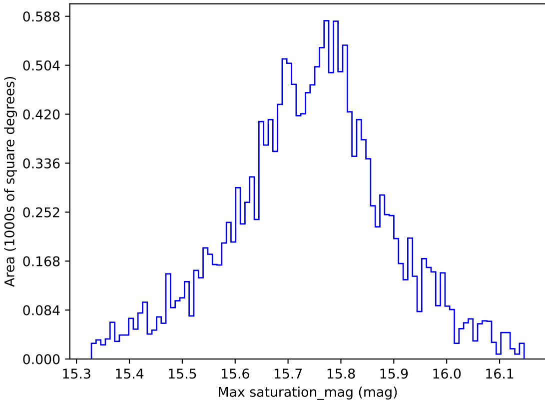
weather_cloudso14v3.4_10yrs WFD r band: Max saturation_mag
