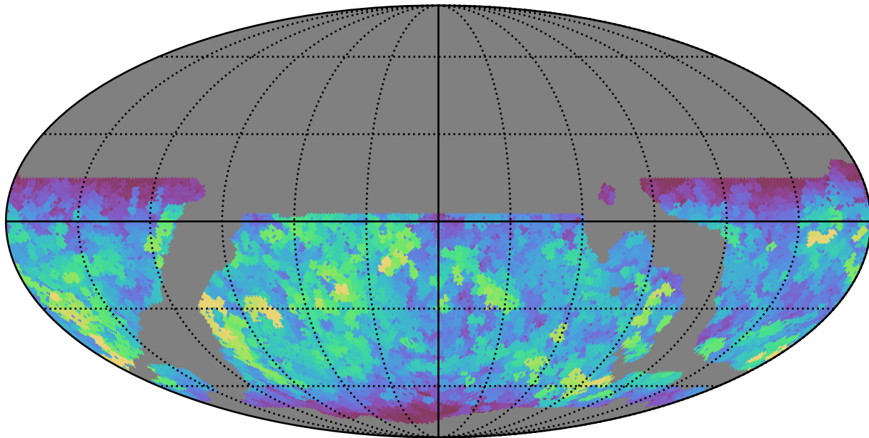
weather_cloudso14v3.4_10yrs WFD i band: Max saturation_mag
