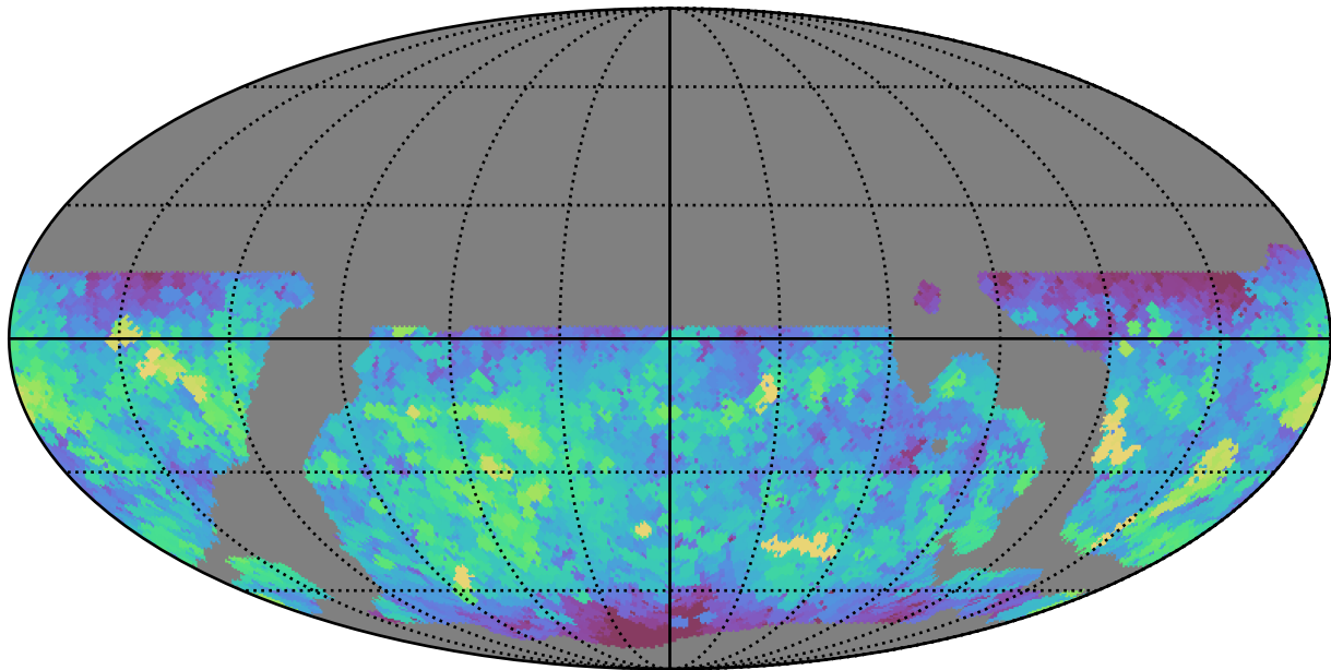
weather_cloudso14v3.4_10yrs WFD g band: Max saturation_mag
