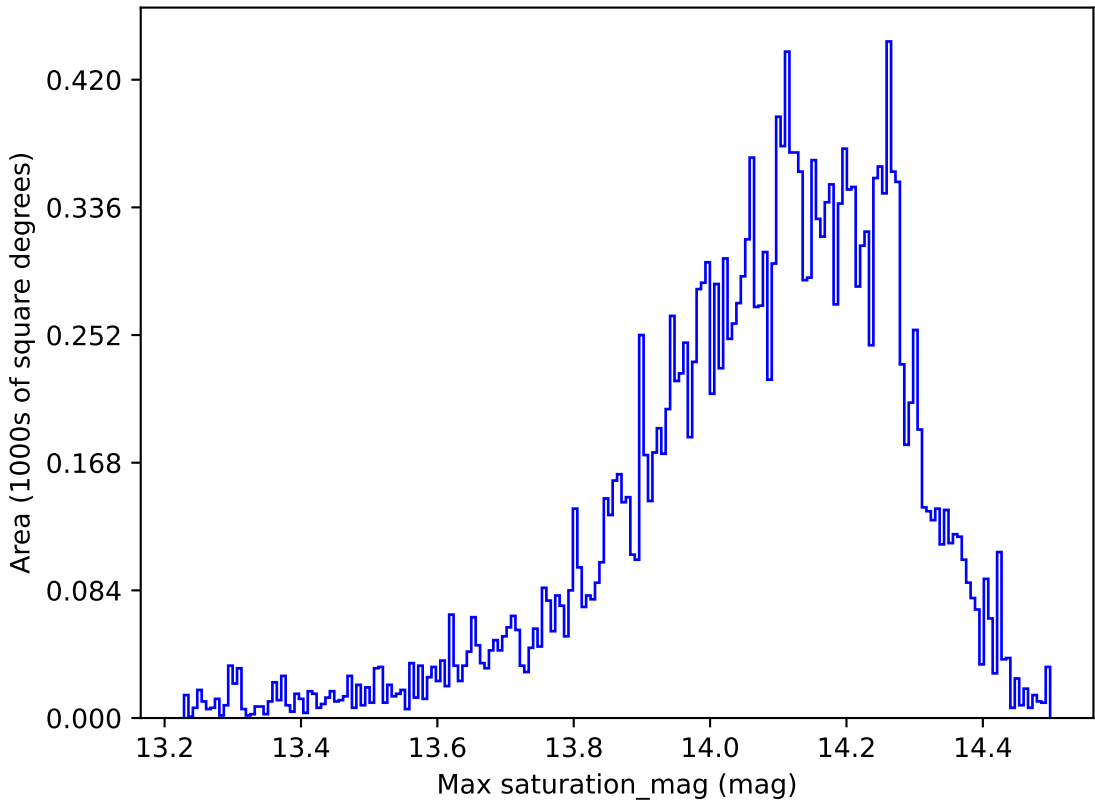
weather_cloudso14v3.4_10yrs All sky y band: Max saturation_mag
