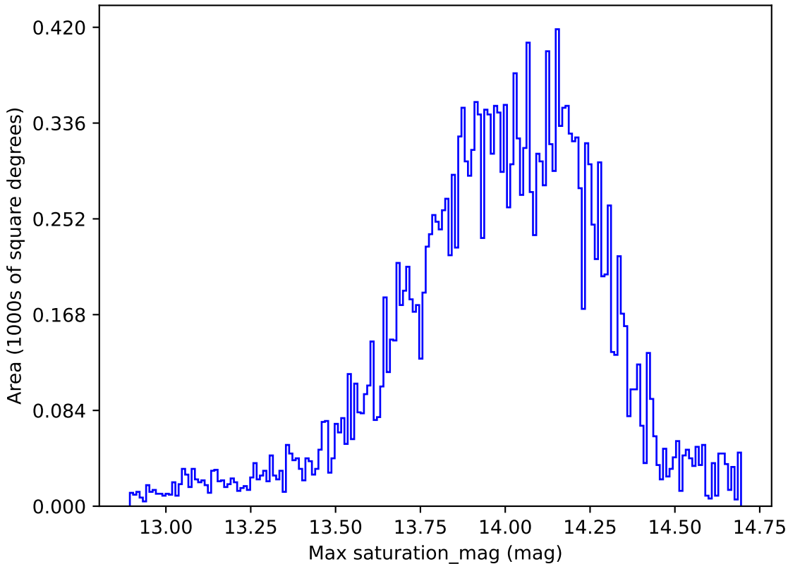
weather_cloudso14v3.4_10yrs All sky u band: Max saturation_mag
