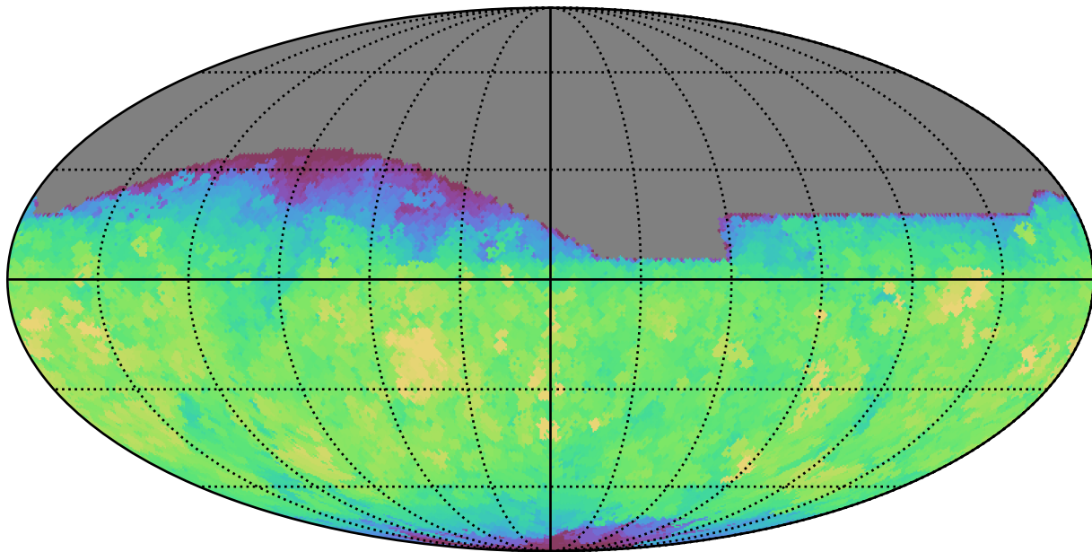
weather_cloudso14v3.4_10yrs All sky r band: Max saturation_mag
