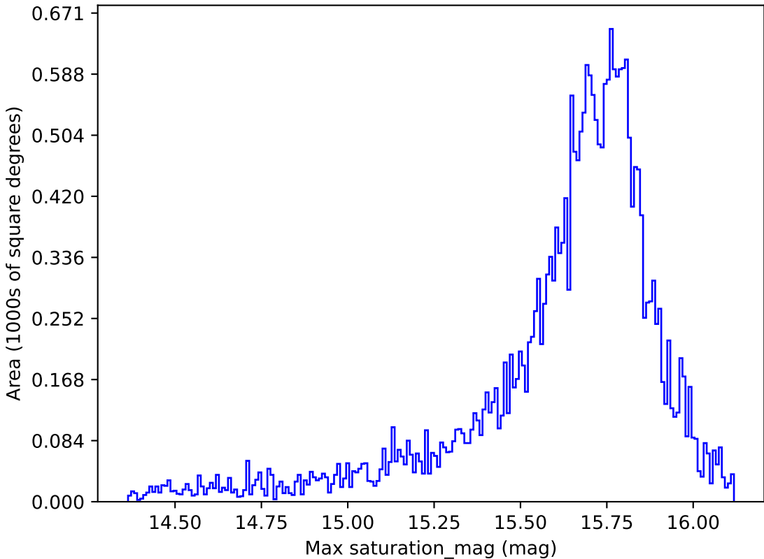
weather_cloudso14v3.4_10yrs All sky r band: Max saturation_mag
