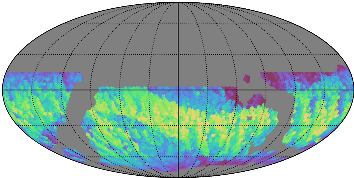
weather_cloudso14v3.4_10yrs WFD z band: Max normairmass
