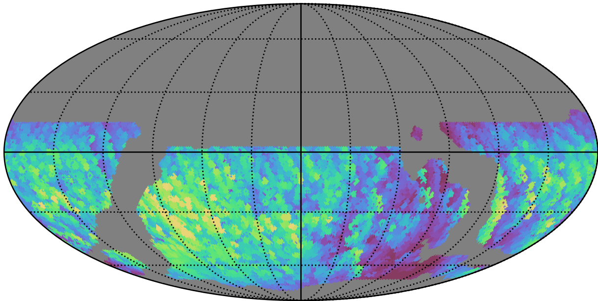
weather_cloudso14v3.4_10yrs WFD y band: Max normairmass
