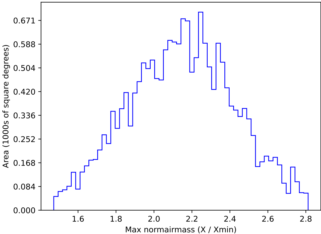
weather_cloudso14v3.4_10yrs WFD y band: Max normairmass
