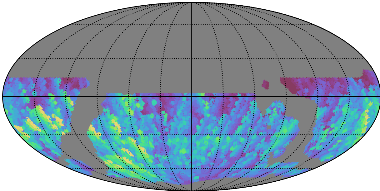
weather_cloudso14v3.4_10yrs WFD g band: Max normairmass
