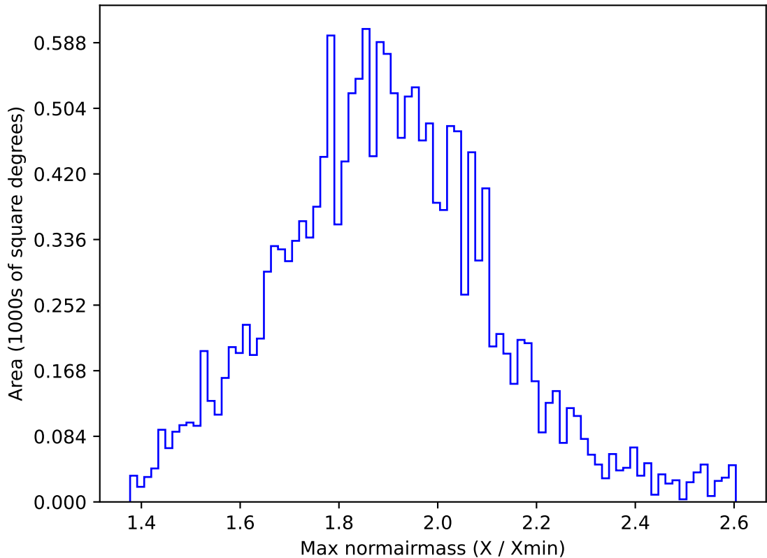
weather_cloudso14v3.4_10yrs WFD g band: Max normairmass
