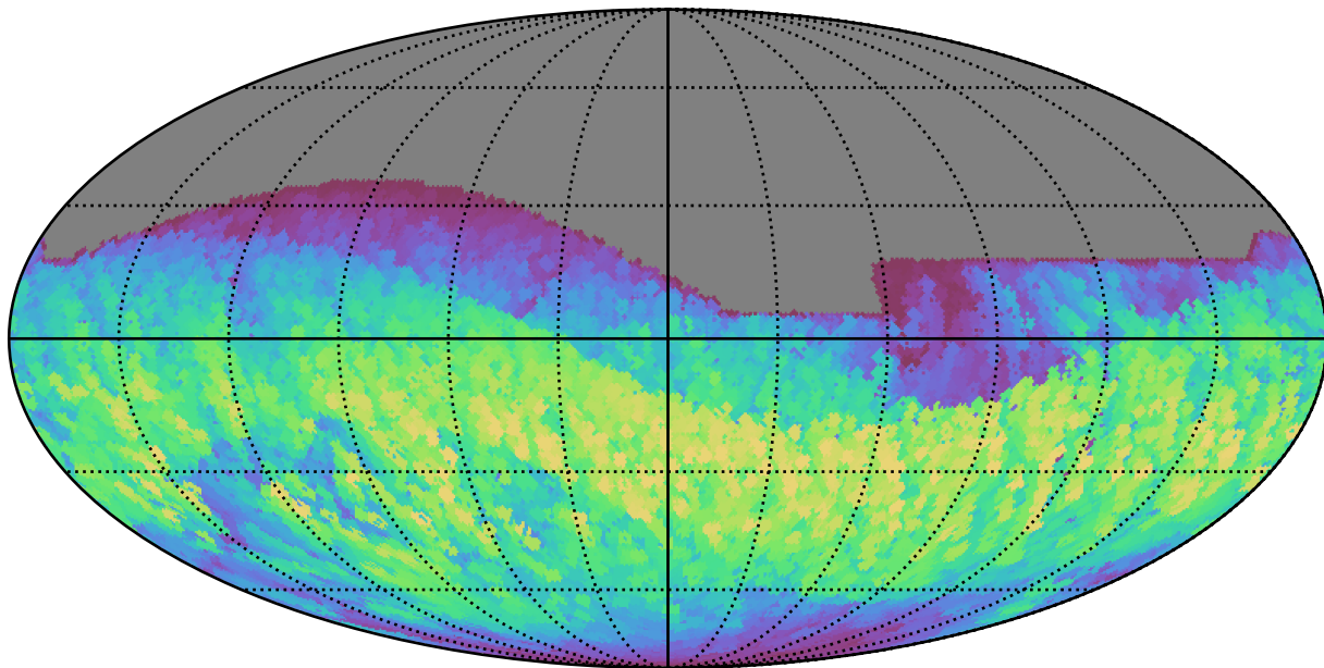
weather_cloudso14v3.4_10yrs All sky i band: Max normairmass
