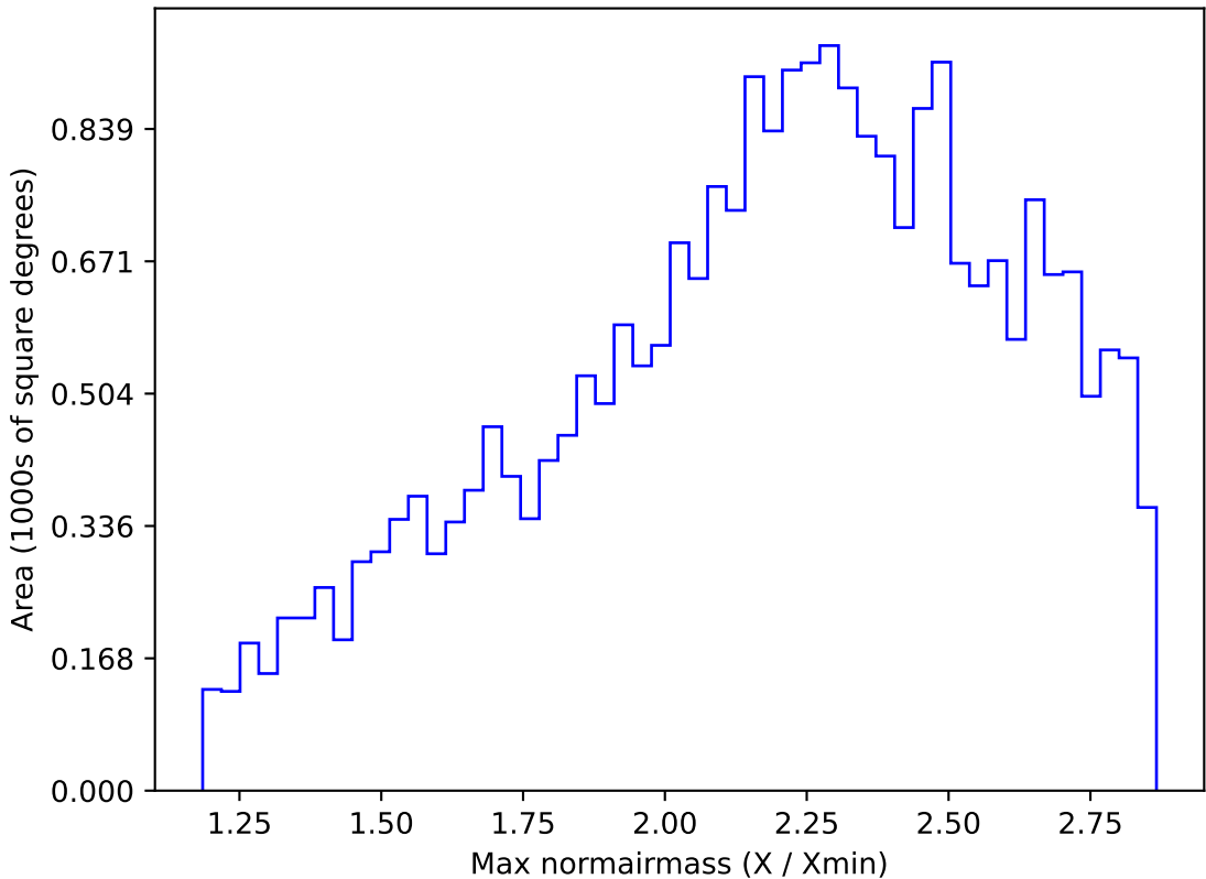
weather_cloudso14v3.4_10yrs All sky i band: Max normairmass
