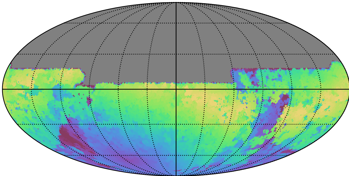
weather_cloudso14v3.4_10yrs All sky y band: Max moonDistance
