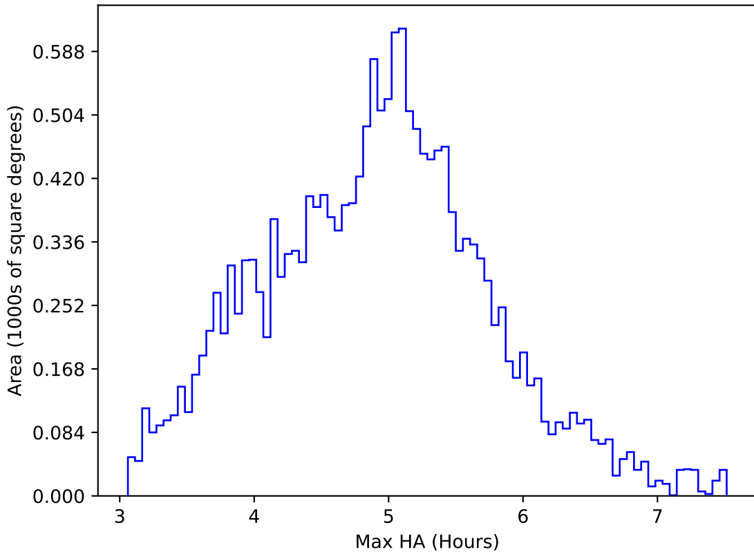
weather_cloudso14v3.4_10yrs WFD z band: Max HA
