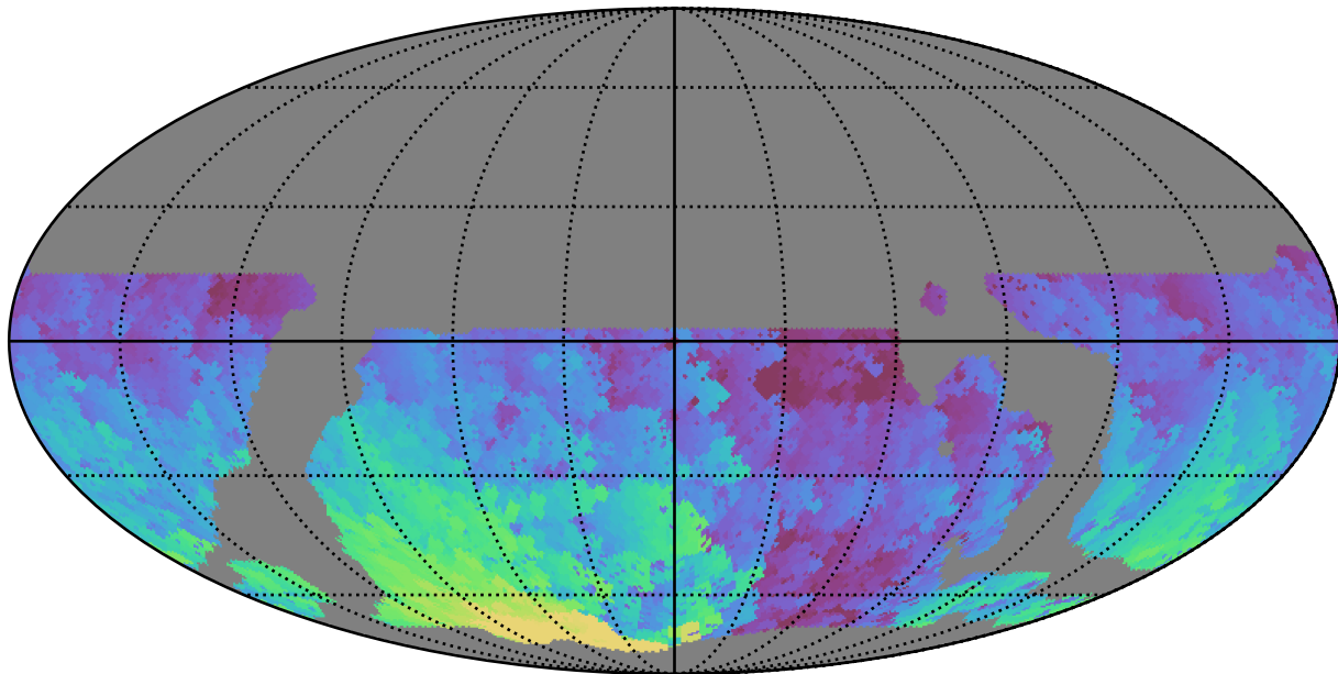
weather_cloudso14v3.4_10yrs WFD u band: Max HA
