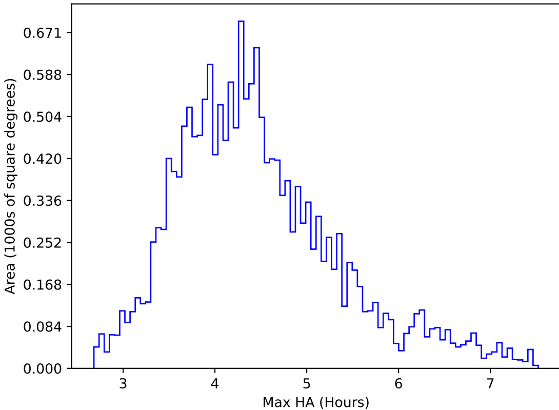
weather_cloudso14v3.4_10yrs WFD r band: Max HA
