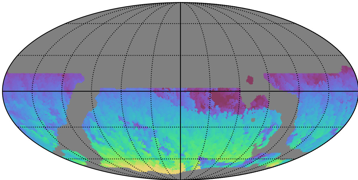
weather_cloudso14v3.4_10yrs WFD i band: Max HA
