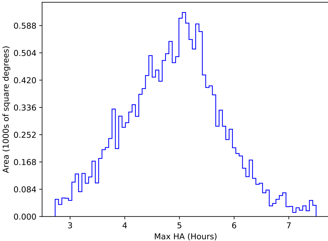
weather_cloudso14v3.4_10yrs WFD i band: Max HA
