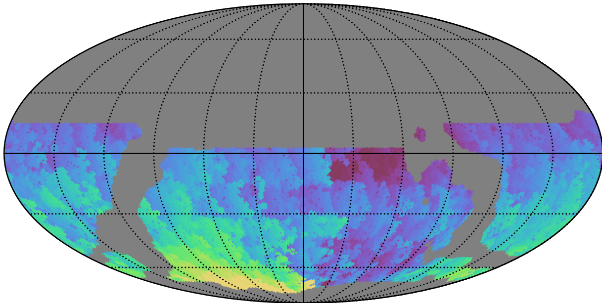
weather_cloudso14v3.4_10yrs WFD g band: Max HA
