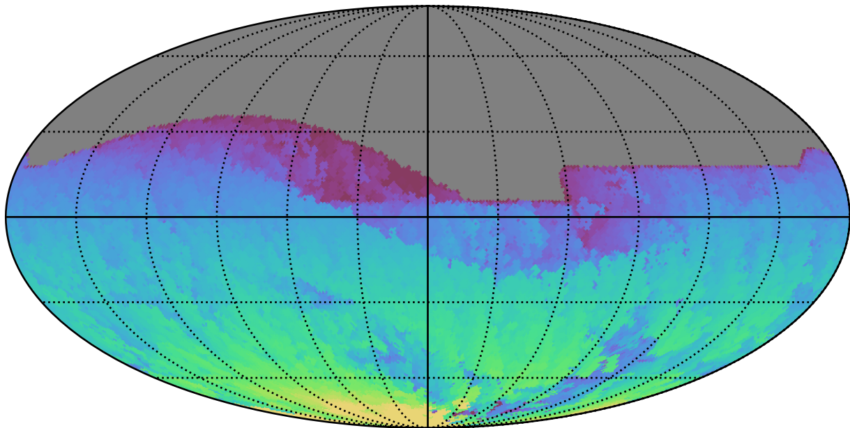
weather_cloudso14v3.4_10yrs All sky z band: Max HA
