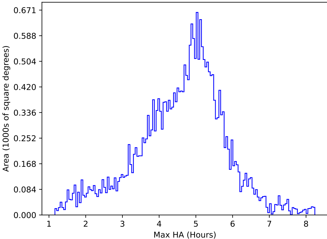
weather_cloudso14v3.4_10yrs All sky z band: Max HA
