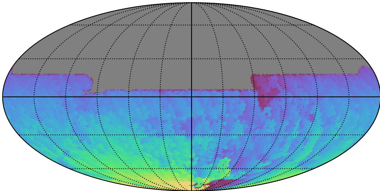
weather_cloudso14v3.4_10yrs All sky y band: Max HA
