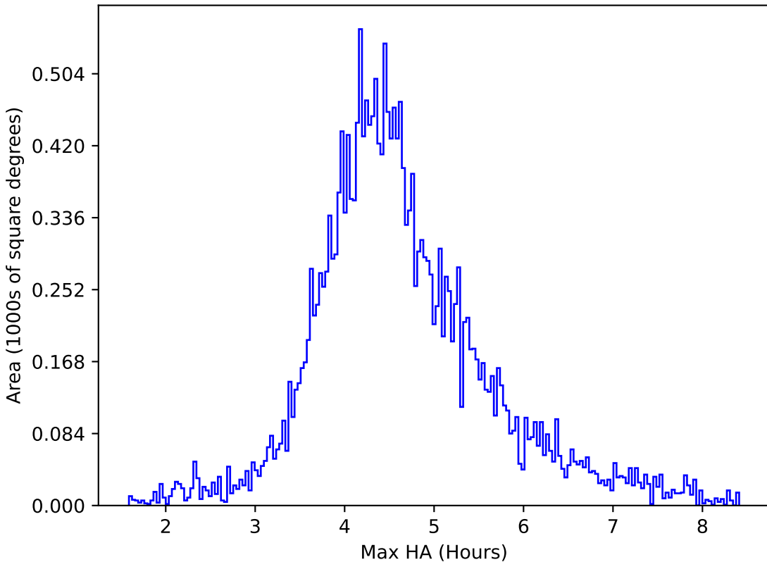
weather_cloudso14v3.4_10yrs All sky y band: Max HA
